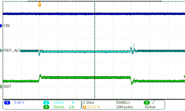
V_{OUT} = 4.2\text{ V} I_{SYS} = 0\text{ mA} \rightarrow 500\text{ mA} \rightarrow 0\text{ mA} I_{CHG} = 250\text{ mA}
