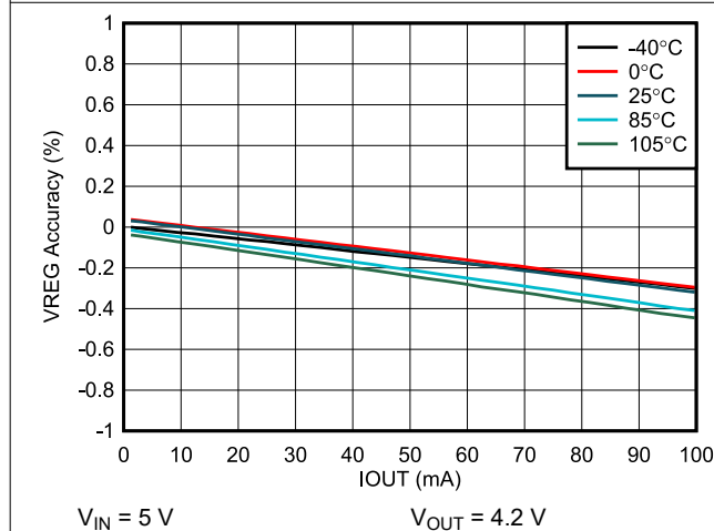
图 6-3. Load Regulation
