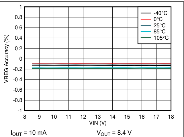
图 6-2. Line Regulation
