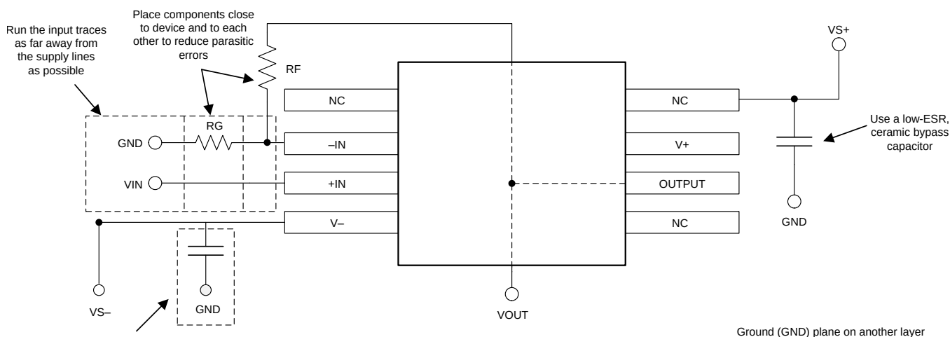
Figure 45. 同相配置的运算放大器电路板布局
