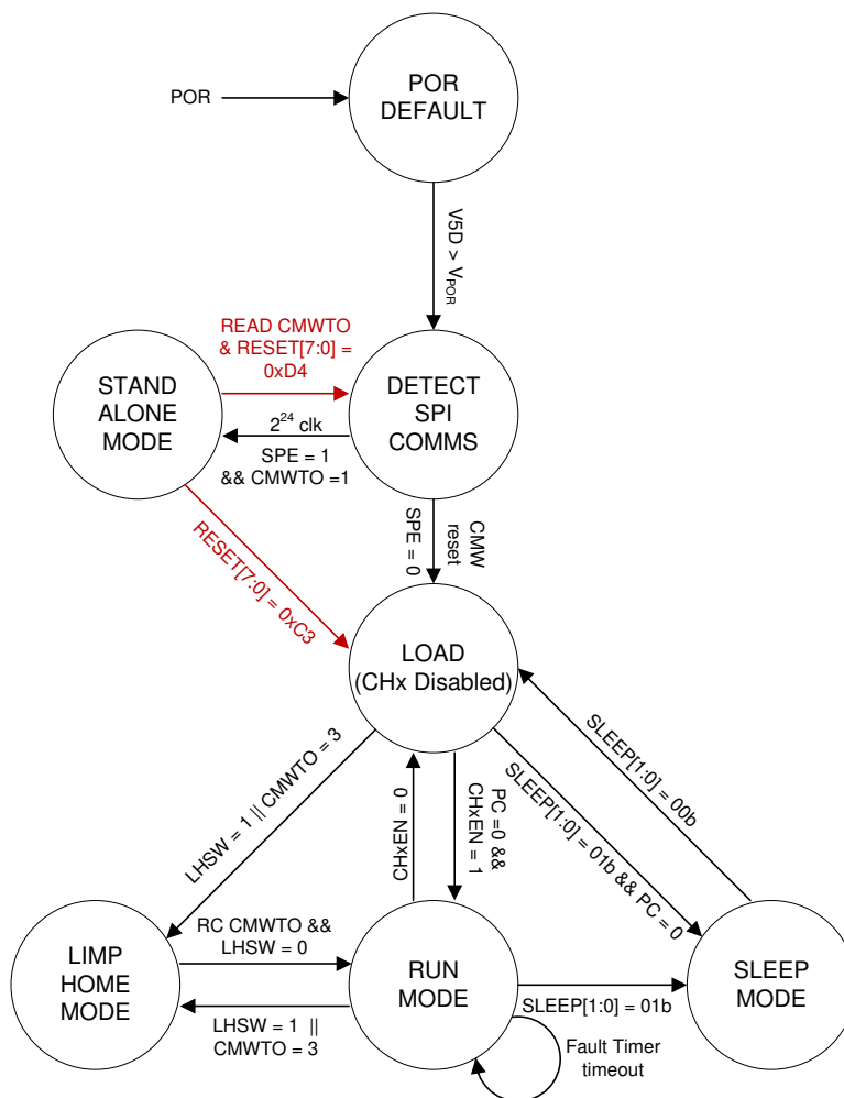
图 7-13. TPS92520-Q1 Functional Modes
