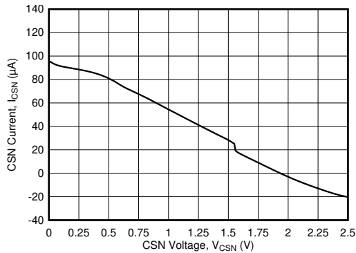
图 6-3. CSN Source Current vs CSN Voltage
