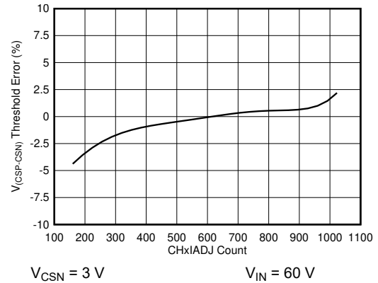
图 6-2. V_{(CSP - CSN)} Current Sense Error vs IADJ Count
