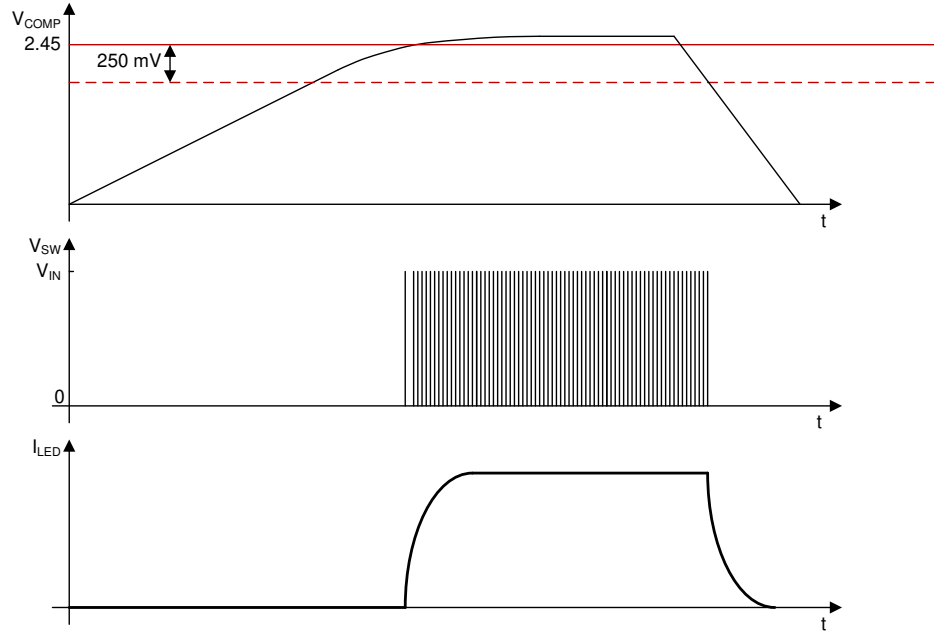
图 7-3. Soft-Start Sequence
