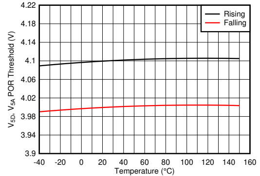
图 6-6. V_{5D,A} POR Threshold vs Temperature
