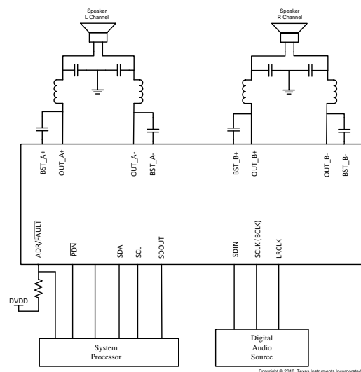
简化方框图
