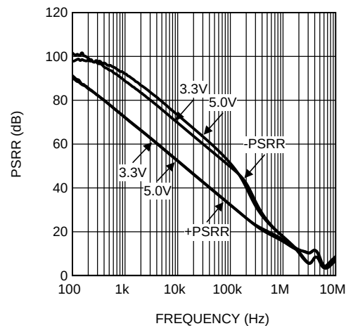
Figure 26. PSRR 与频率间的关系
