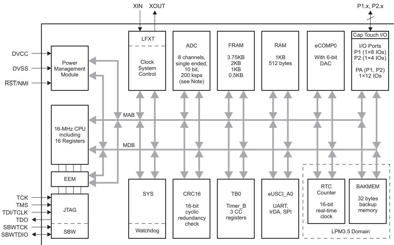
图 1-1. 功能框图
