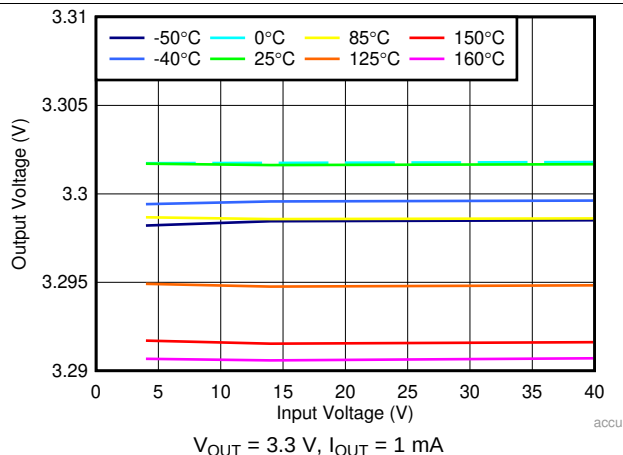
图 13. Output Voltage vs Input Voltage
