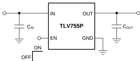
典型应用
