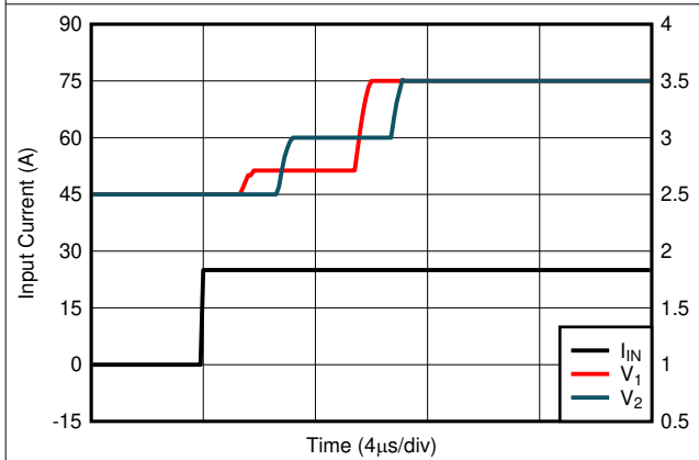
图 7-9. Voltage Output Step, Rising
