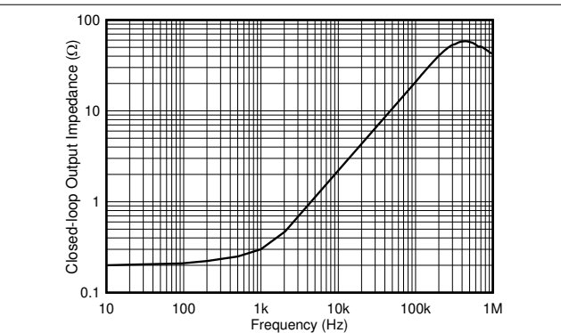
图 7-6. Output Impedance vs. Frequency
