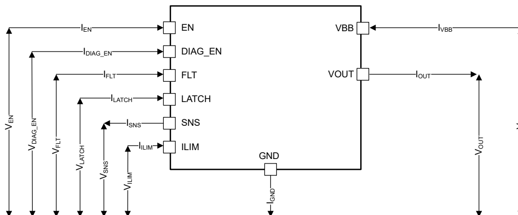
图 7-1. Parameter Definitions
