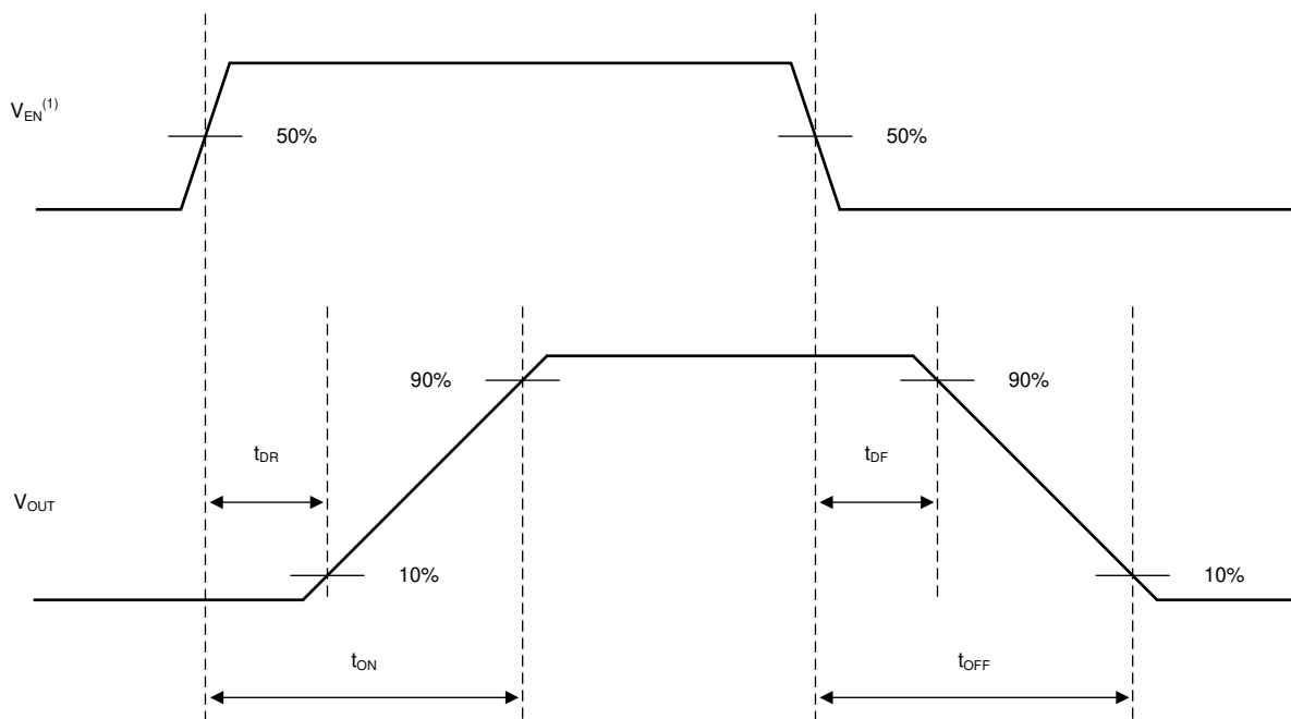
图 7-1. Parameter Definitions
