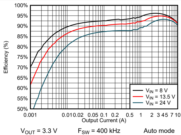
图 9-7. Efficiency
