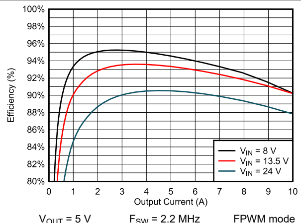
图 9-10. Efficiency
