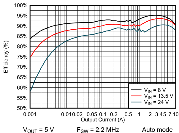
图 9-9. Efficiency
