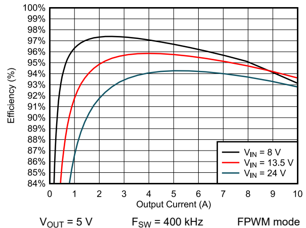
图 9-6. Efficiency
