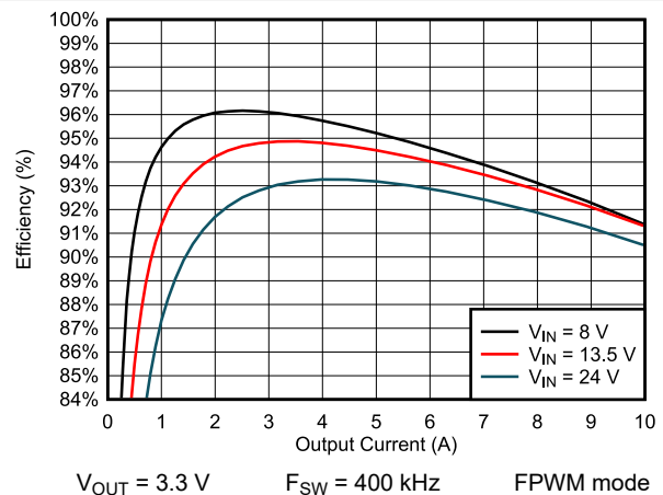
图 9-8. Efficiency
