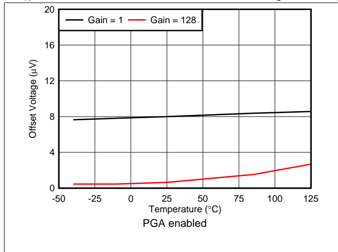
图 16. Input Offset Voltage vs Temperature
