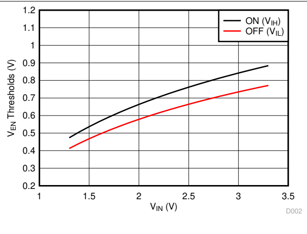
图 6-2. V_{EN} Thresholds vs V_{IN}
