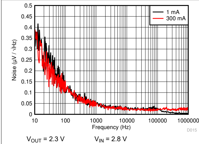
图 6-15. Noise Density
