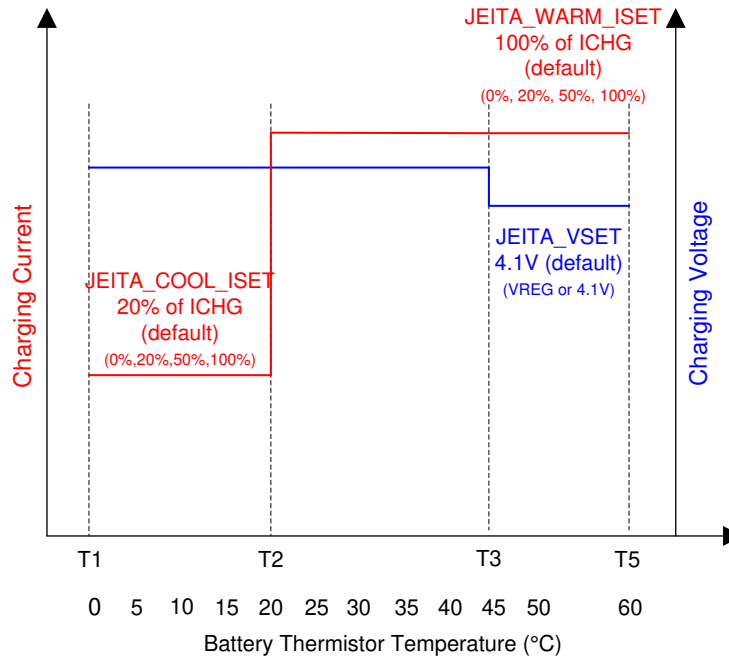
图 14. JEITA Profile
