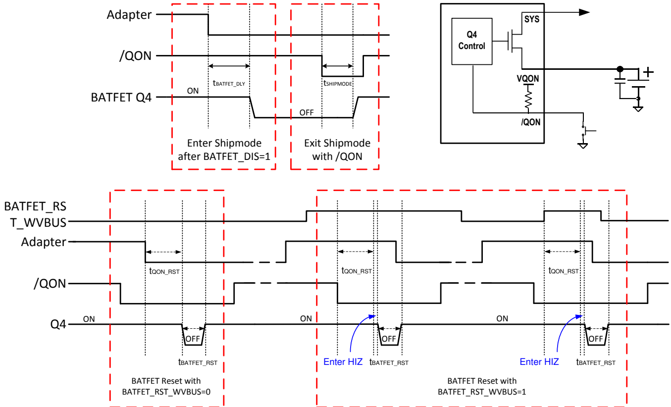
图 16. \overline{QON} Timing
