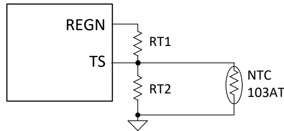
图 15. TS Pin Resistor Network
