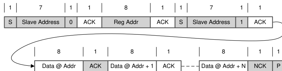
图 24. Multi-Read
