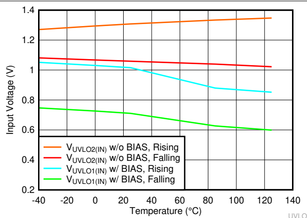
图 7-37. V_{IN} UVLO vs Temperature
