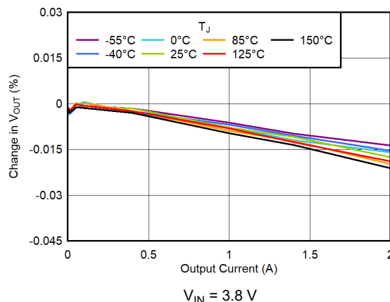
图 7-52. Load Regulation (3.3-V Output)
