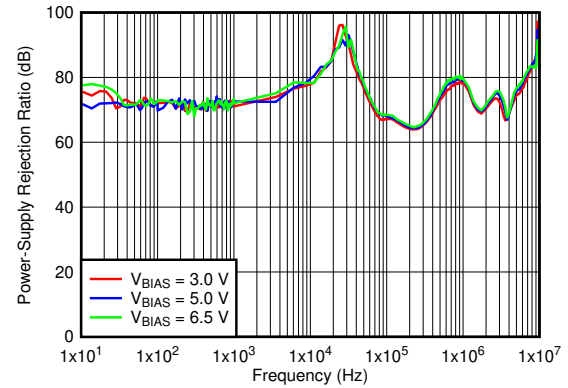
图 7-8. V_{BIAS} PSRR vs Frequency
