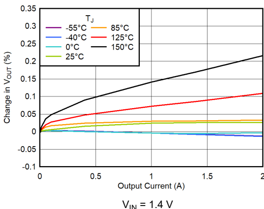
图 7-51. Load Regulation
