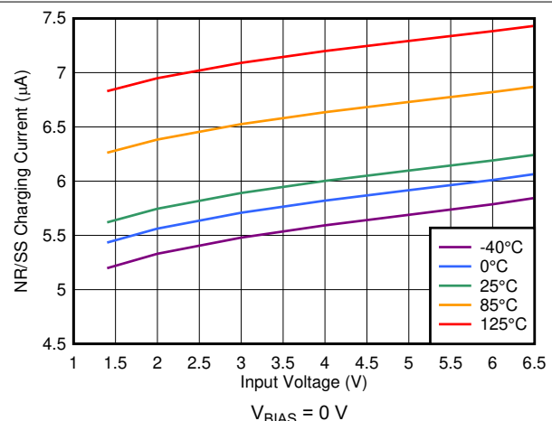
图 7-36. I_{NR/SS} Current vs Input Voltage
