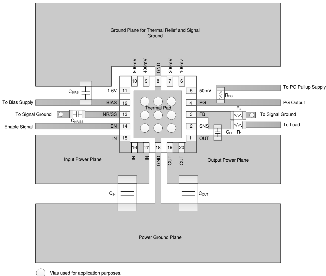
图 11-1. Example Layout
