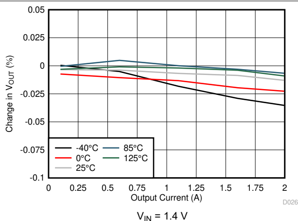
图 7-26. Load Regulation
