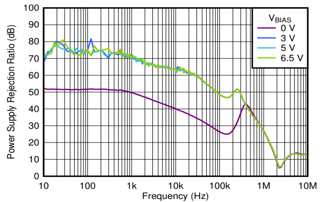
图 7-44. PSRR vs Frequency and V_{BIAS}
