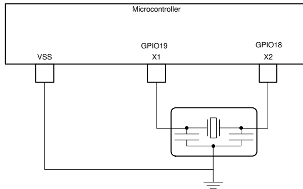
图 7-14. External Resonator
