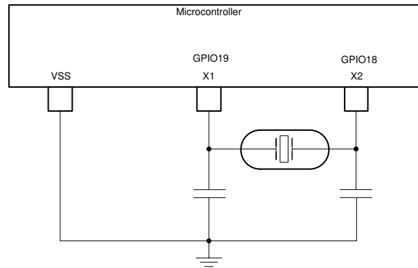
图 7-13. External Crystal
