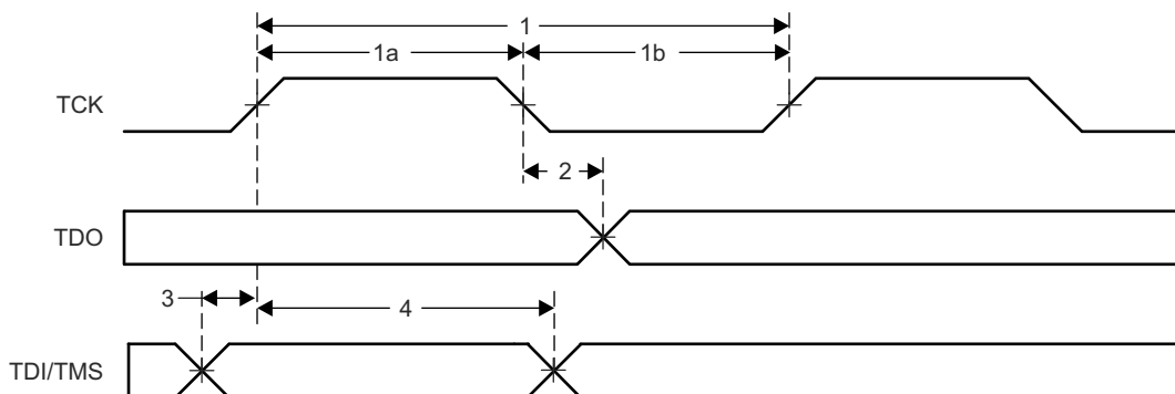
图 7-19. JTAG Timing
