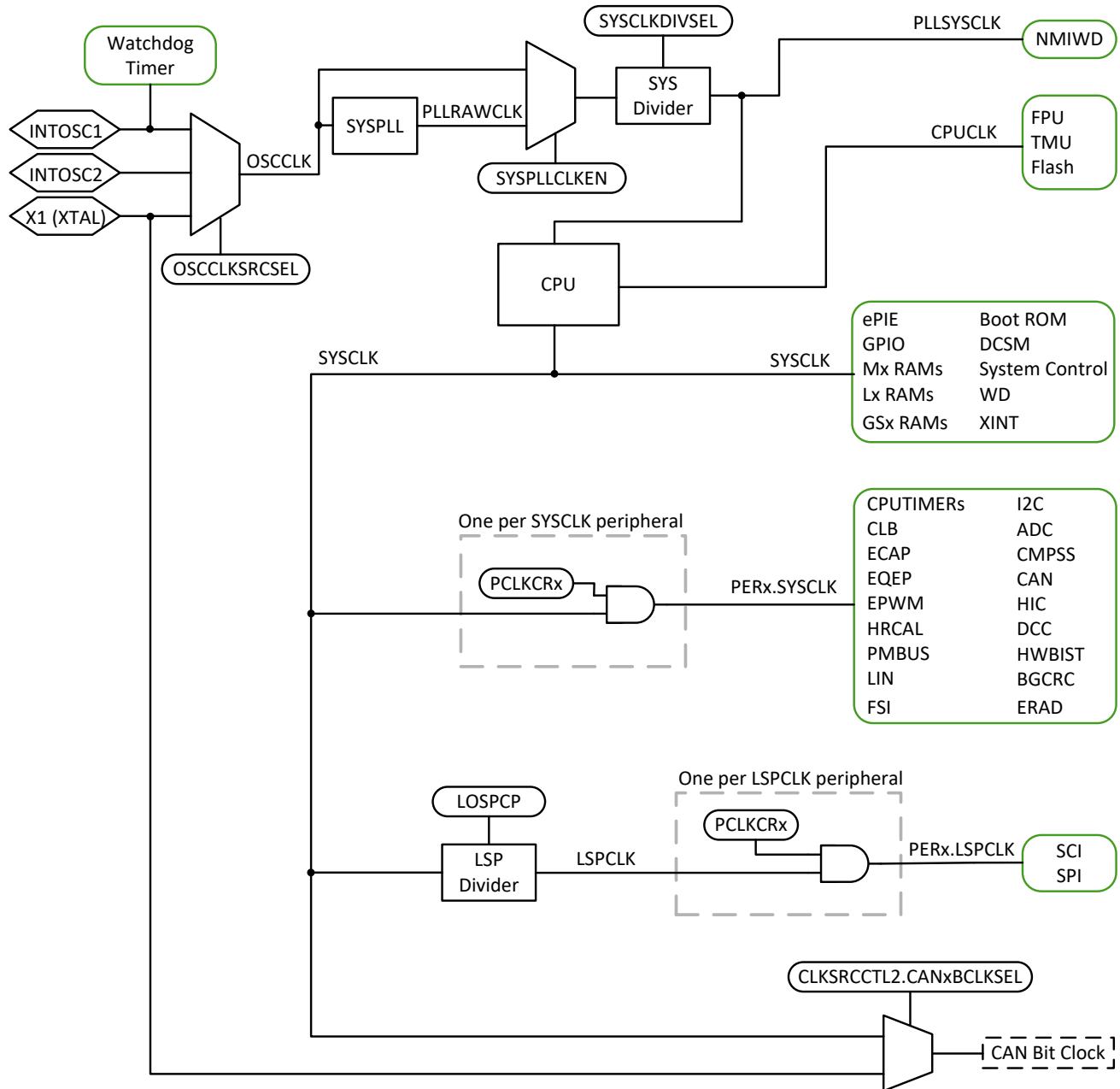
图 7-10. Clocking System
