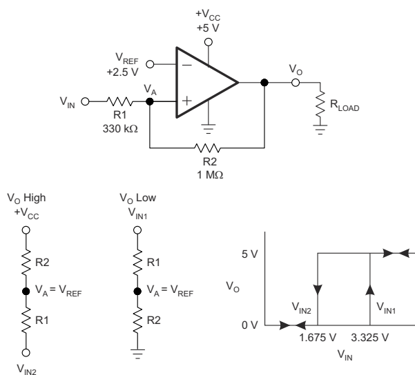
图 8-2. TLV703x-Q1 在具有迟滞的非反相配置中
