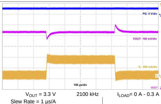
图 39. Load Transient
