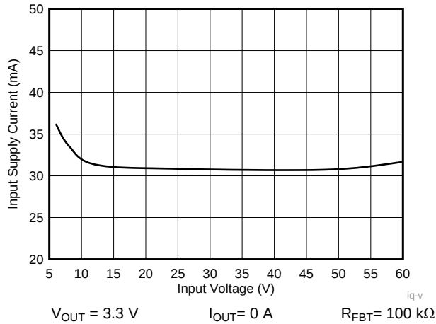
图 28. Input Supply Current
