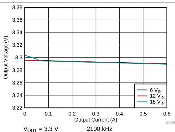
图 35. Load Regulation
