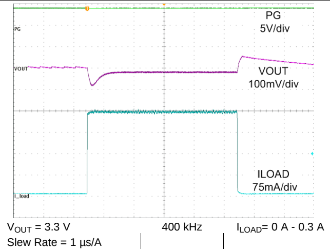
图 33. Load Transient
