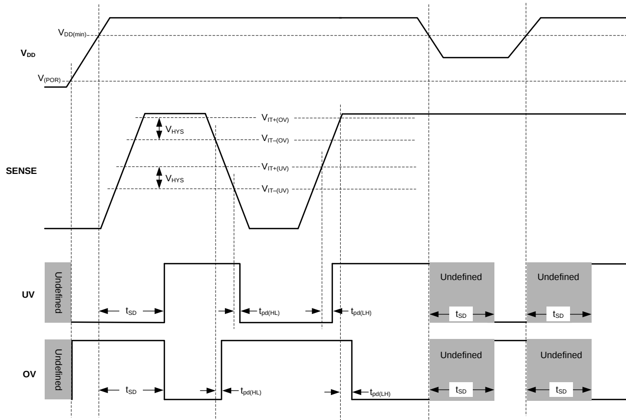
图 1. Timing Diagram
