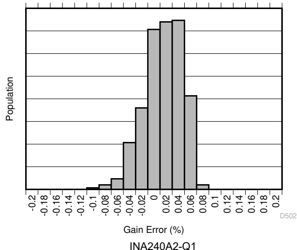
图 7-6. Gain Error Production Distribution
