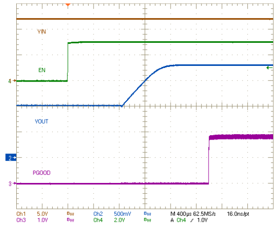
图 52. EN Start-up With Prebiased Output
