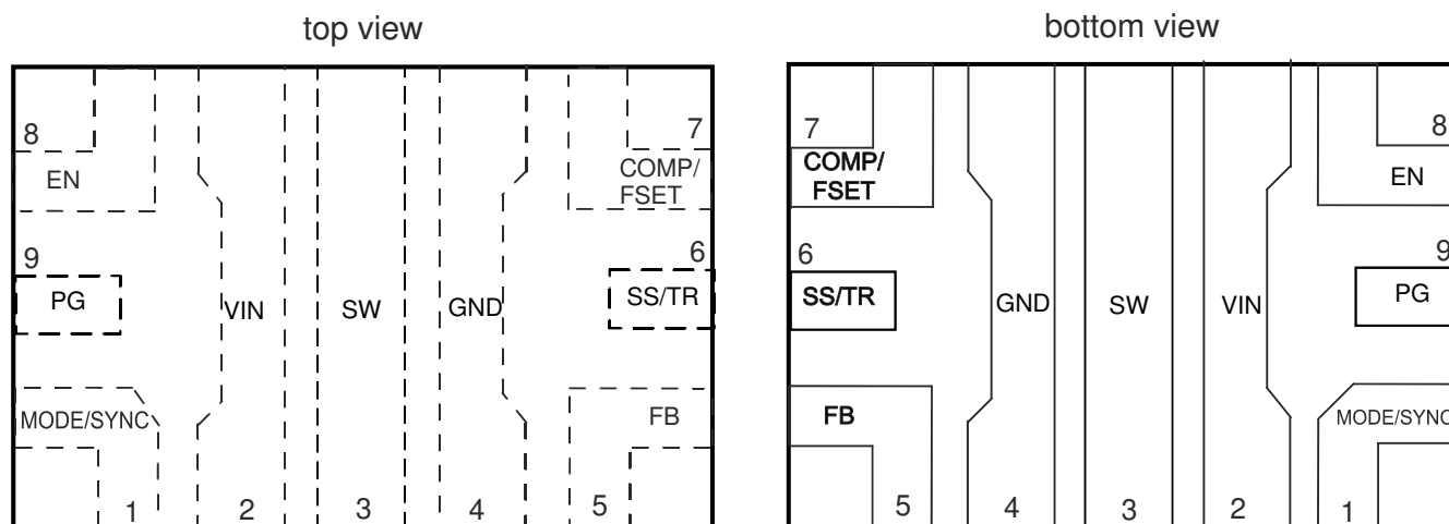
图 6-1. RWY Package 9 Pin (VQFN) Top View
