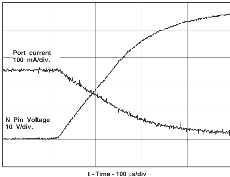
图 8-17. Rdn Function Waveforms
