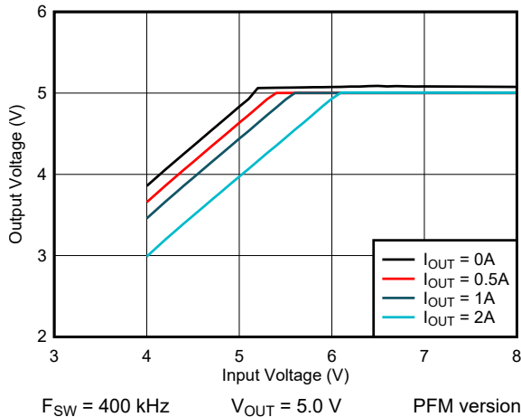
图 7-3. 5-V Dropout
