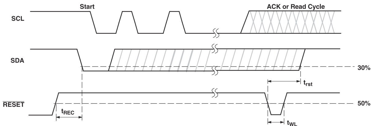
图 7-2. Reset Timing
