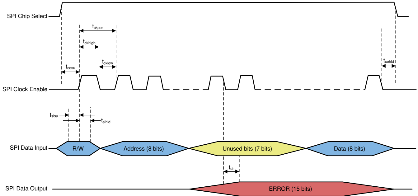
图 7-3. SPI Timing
