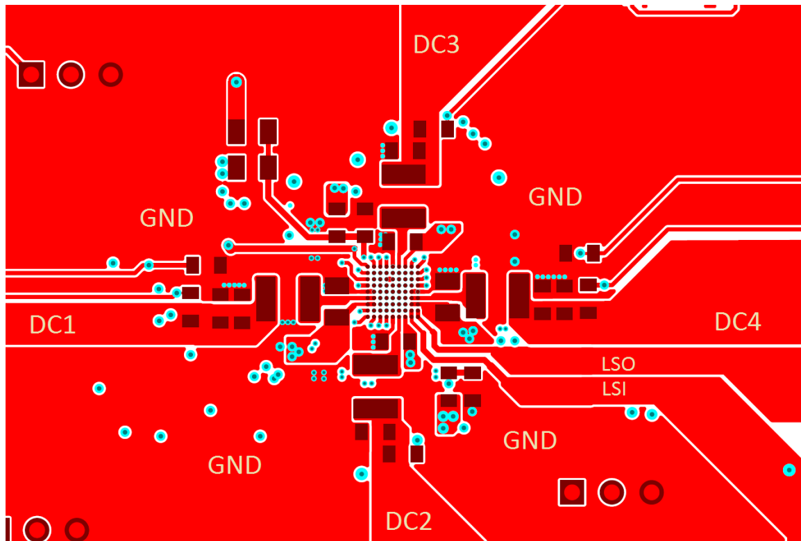
图 10-1. Layout Example
