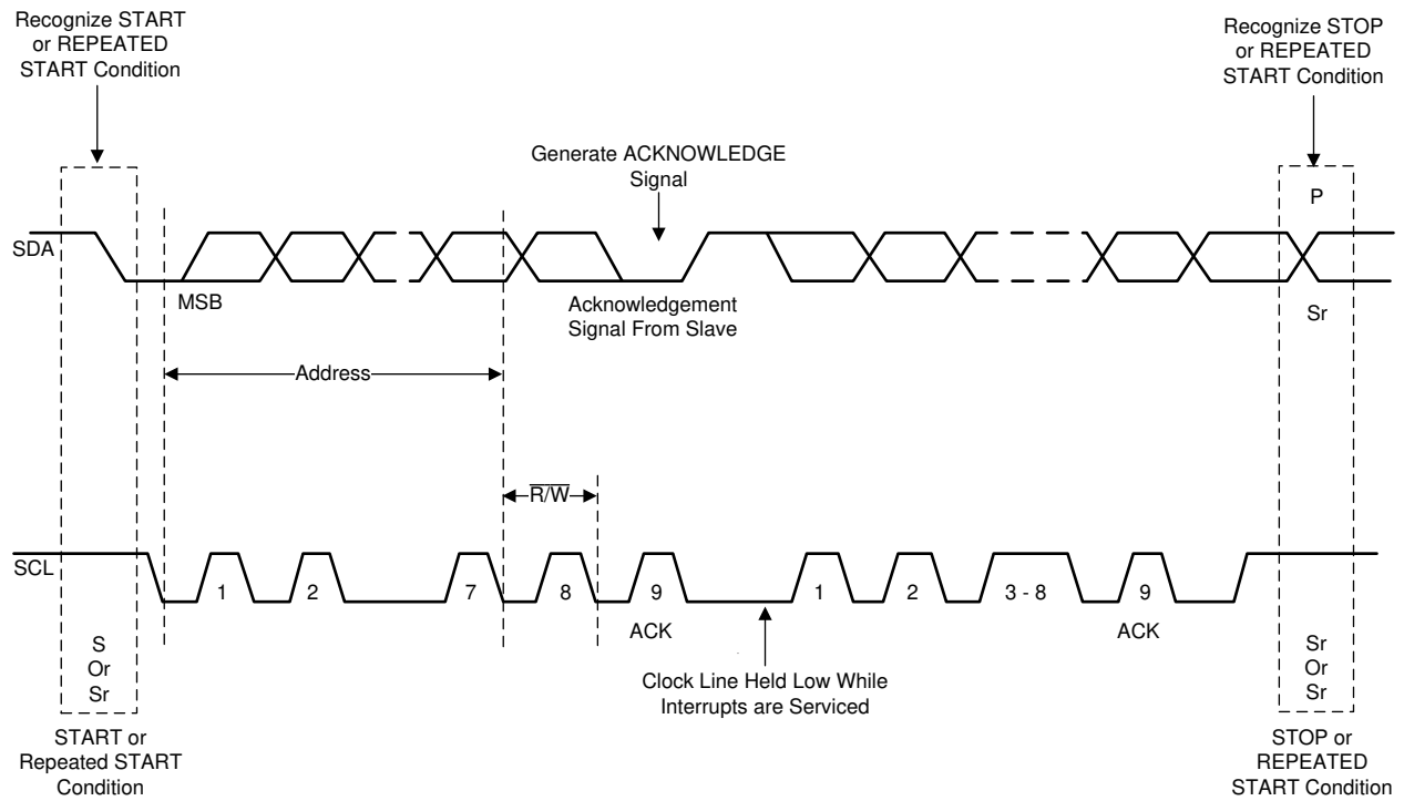
图 8-22. Bus Protocol
