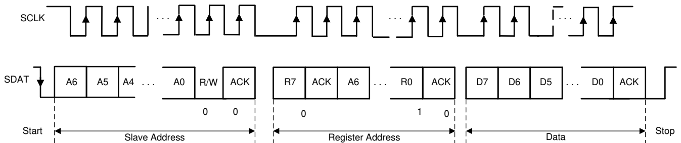
图 8-22. Bus Protocol
