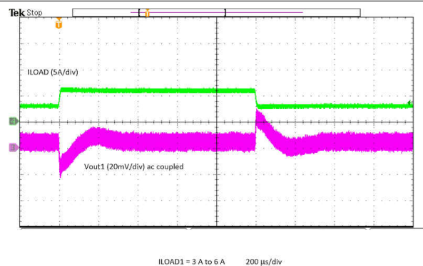
图 8-13. V_{OUT1} Load Transient
