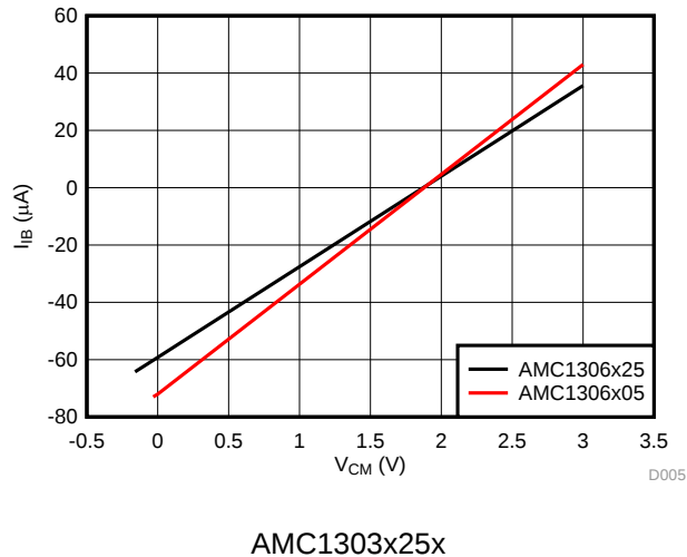
图 56. 输入电流与输入共模电压间的关系
