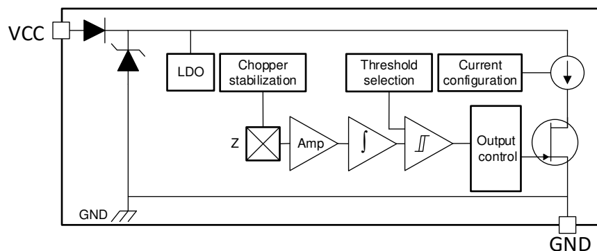
图 8-1. Block Diagram
