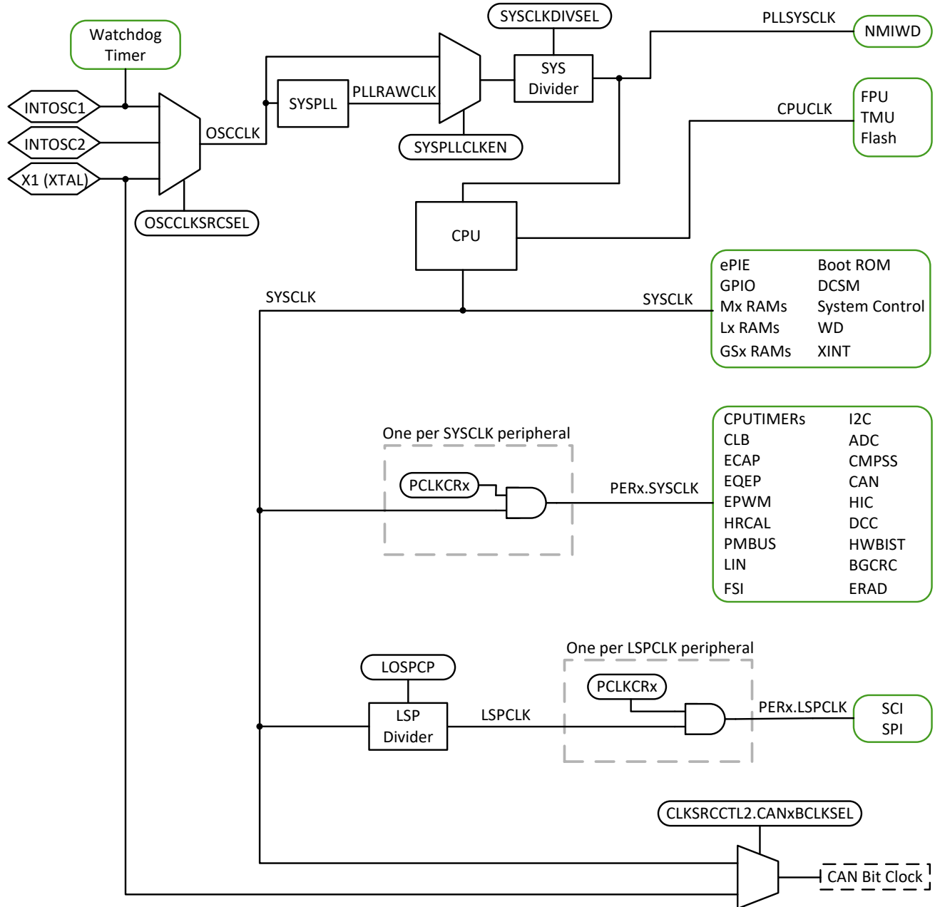
图 7-10. Clocking System
