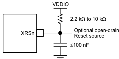
图 7-7. Reset Circuit
