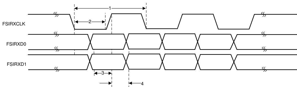
图 7-68. FSIRX Timings
