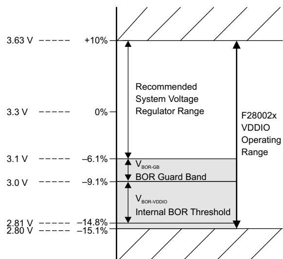
图 7-1. Supply Voltages
