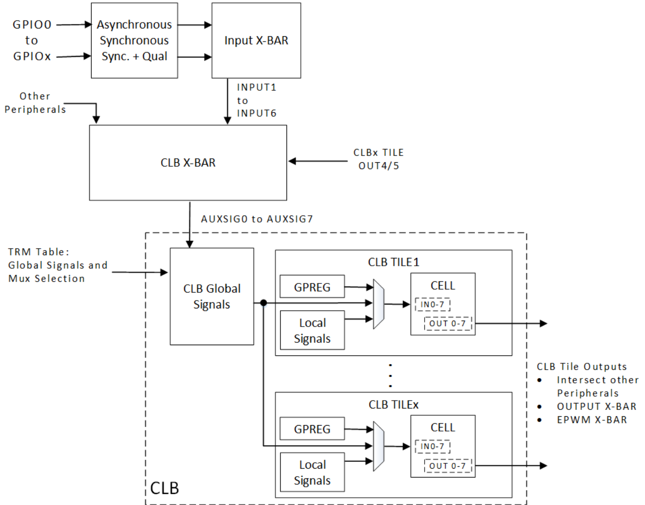
图 8-4. CLB Overview
