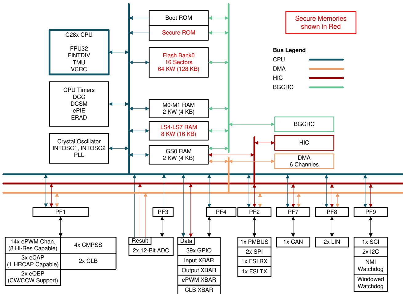
图 3-1. 功能方框图
