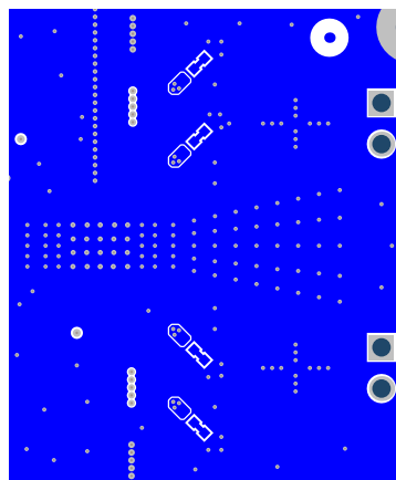
图 54. Layout Example (Stereo) - Bottom Layer
