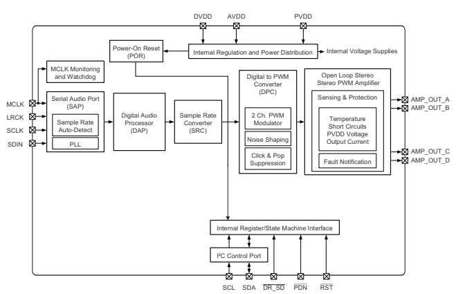
简化框图
