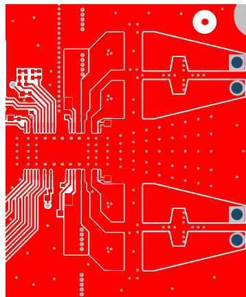
图 53. Layout Example (Stereo) - Top Layer
