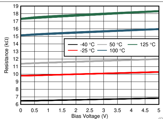
图 6. 电源相关电阻与偏置电压间的关系
