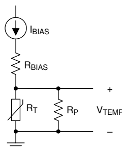
Figure 14. 线性热敏电阻的电流偏置电路
