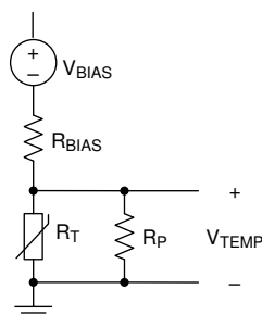
Figure 13. 线性热敏电阻的电压偏置电路
