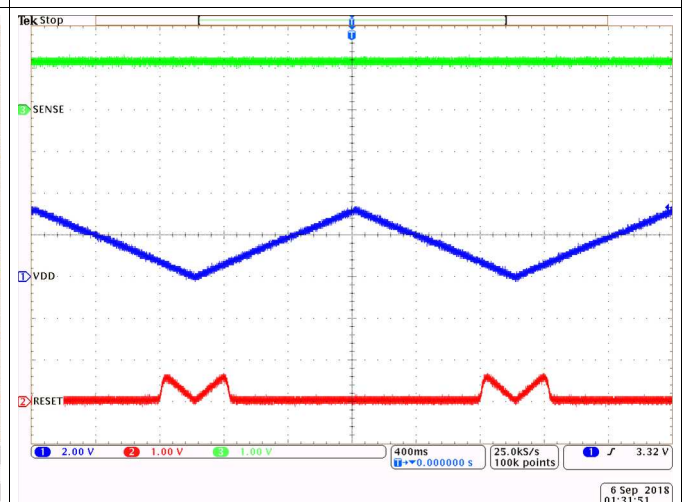
图 37. TPS3703-Q1 CT Bias Unlatch Function
