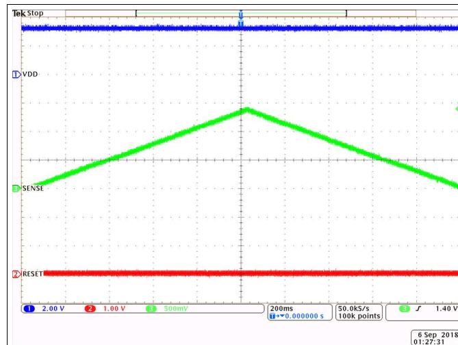
图 36. TPS3703-Q1 SENSE Ramp Latch Function
