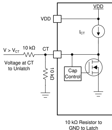
图 27. RESET Latch Circuit
