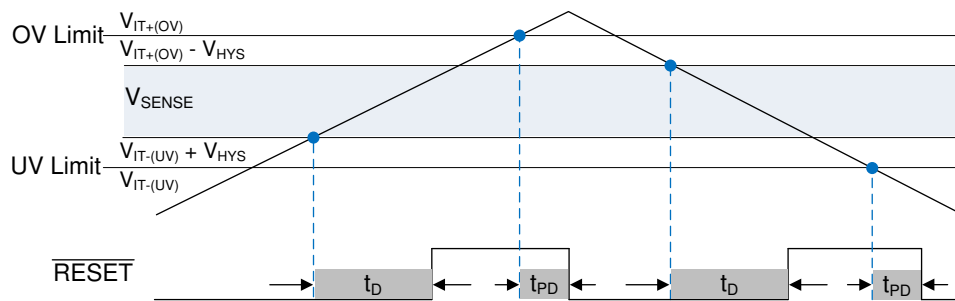
图 23. RESET output
