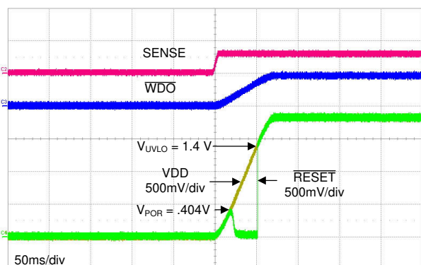
图 8-7. Startup Waveform
