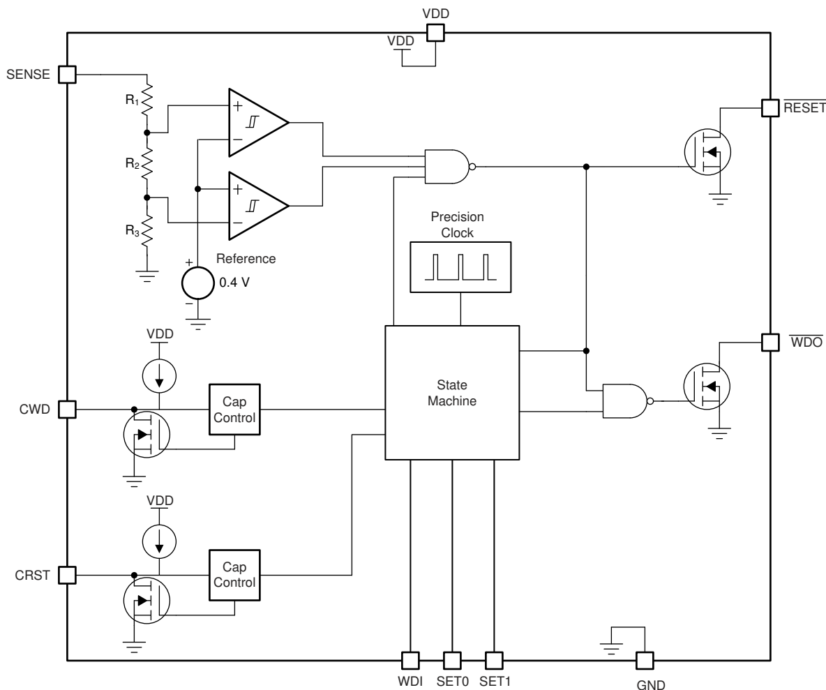
图 7-1. Fixed Version Block Diagram
