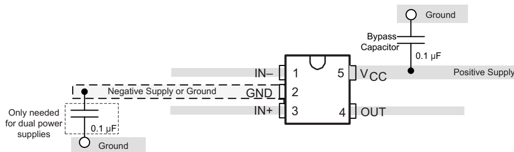
图 10-1. TL331 Layout Example
