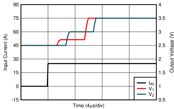
图 7-17. Voltage Output Step, Rising
