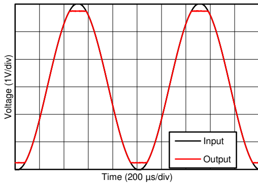
图 8-25. No Phase Reversal
