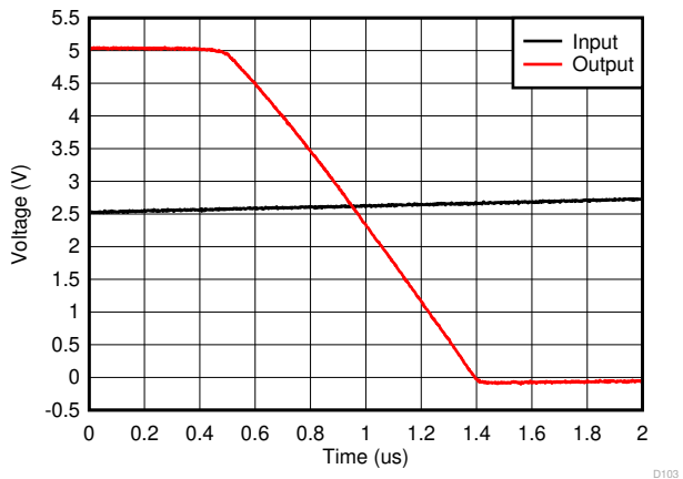
图 10-6. Falling Edge
