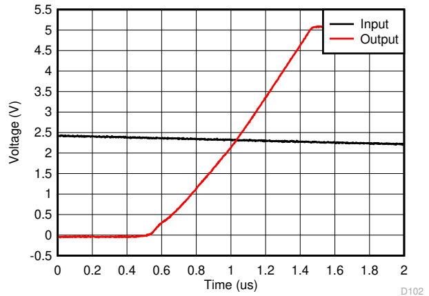
图 10-5. Rising Edge
