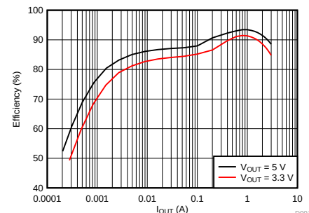
效率与负载间的关系，VIN = 12V，PFM 选项
