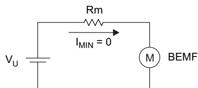
图 35. Mechanical AVS
