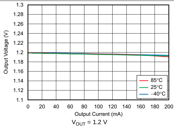
图 1. Load Regulation
