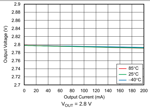
图 2. Load Regulation
