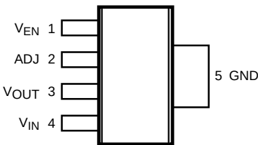
图 1. SOT-223 (LP38692MP-ADJ) - 顶视图 请见封装编号 NDC0005A
