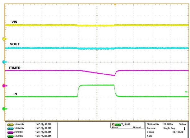
图 9-5. Transient Overload
