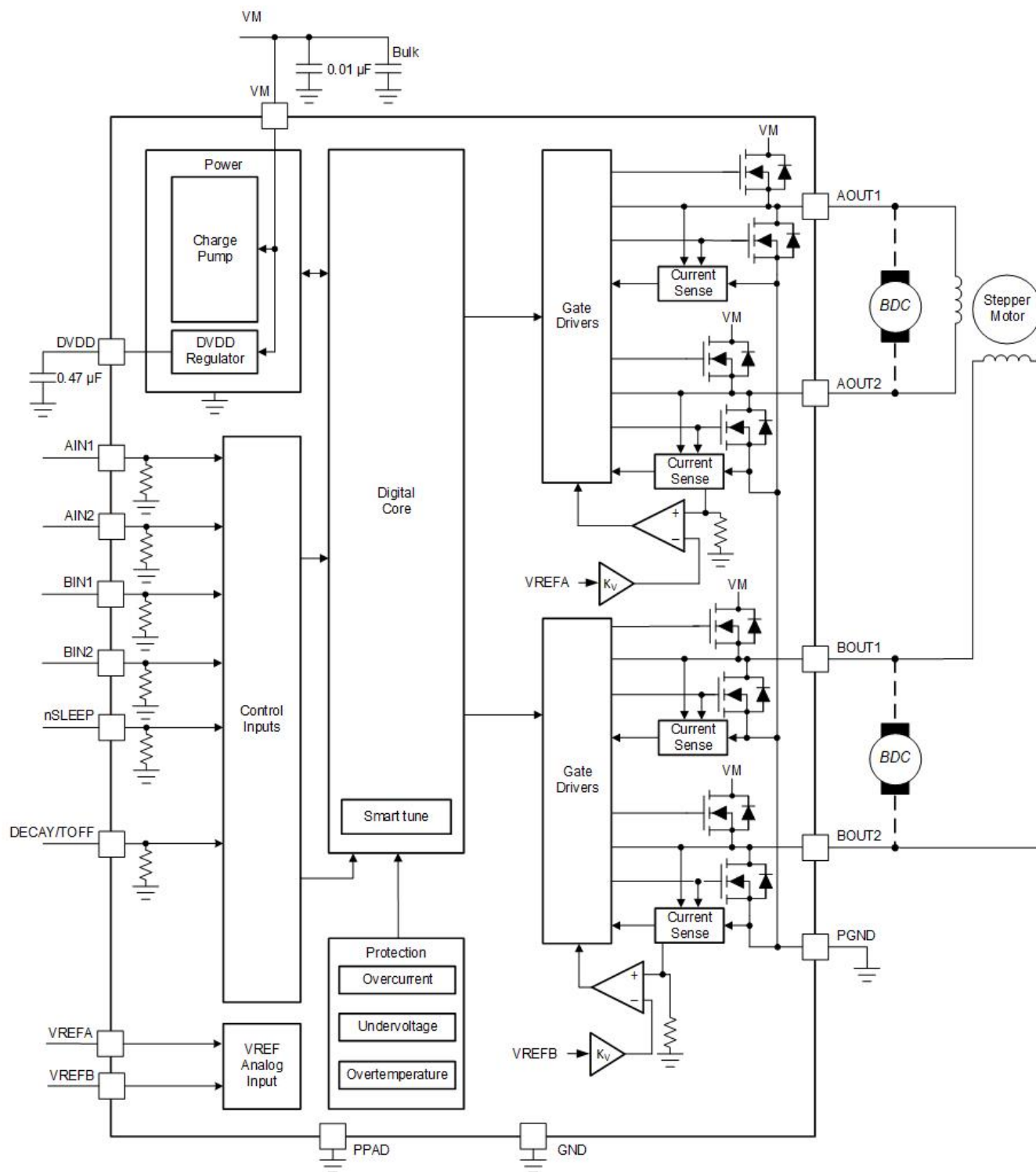
图 7-2. DRV8428P 方框图
