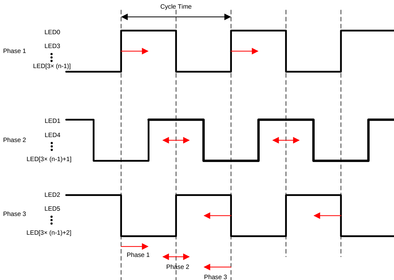
图 12. PWM Phase-Shifting
