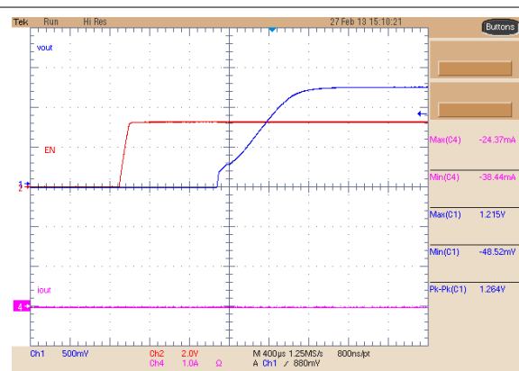
图 8-4. Buck 1 Soft-Start
