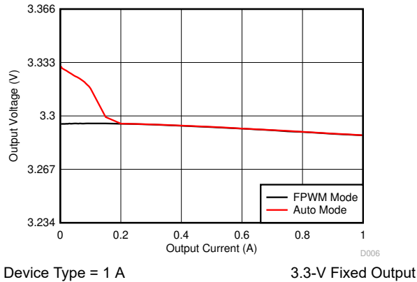
图 9-15. Load Regulation
