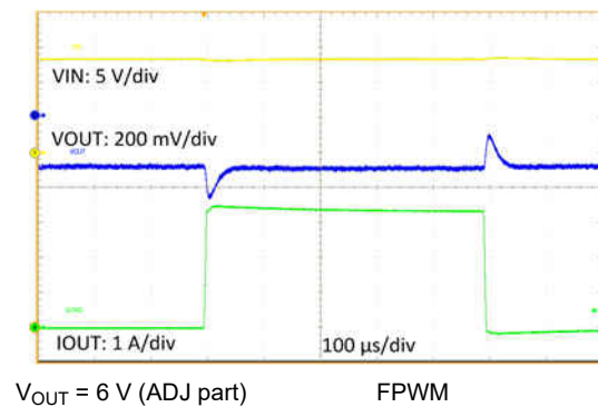
图 9-38. Load Transient
