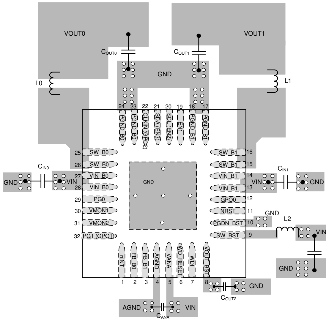
图 10-1. LP87702 Board Layout Example
