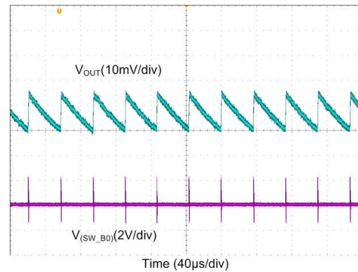
图 8-14. Buck Output Voltage Ripple, PFM Mode
