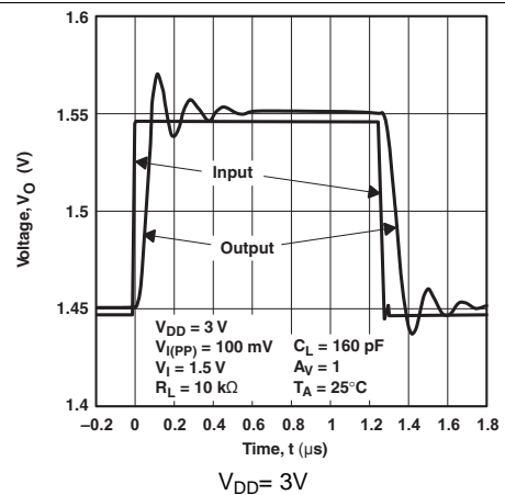
图 42. 小信号跟随器
