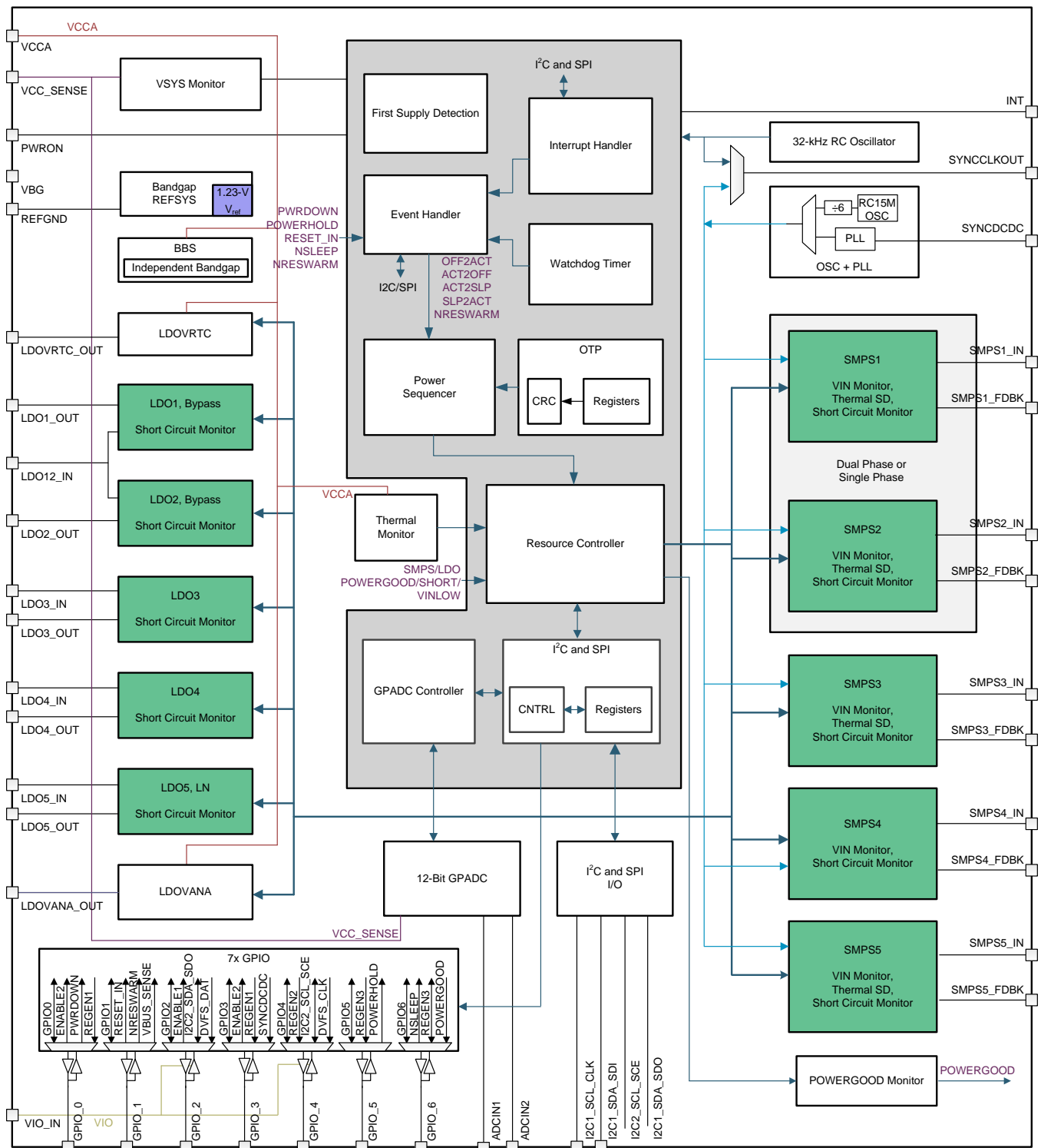
图 1-1. 功能图
